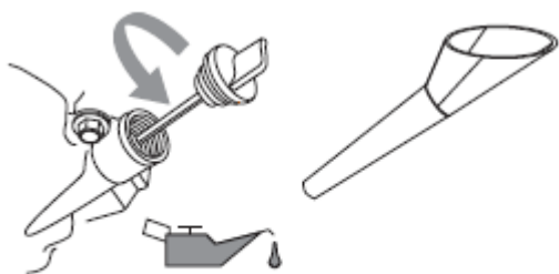
Рисунок -2 Отверстие для заливки масла с воронкой
