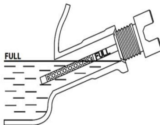
Рисунок-3 Безопасный рабочий диапазон
