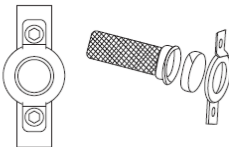
Рисунок-16 Экран искрогасителя
